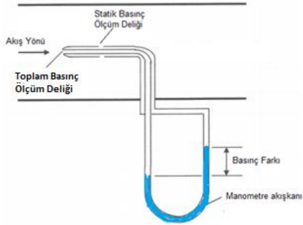
Şema 1: Pitot-Statik basınçölçerin şematik gösterimi
